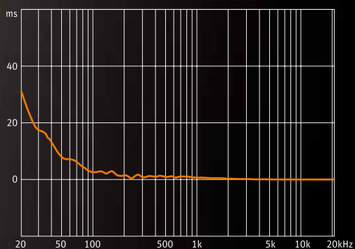
群延时
