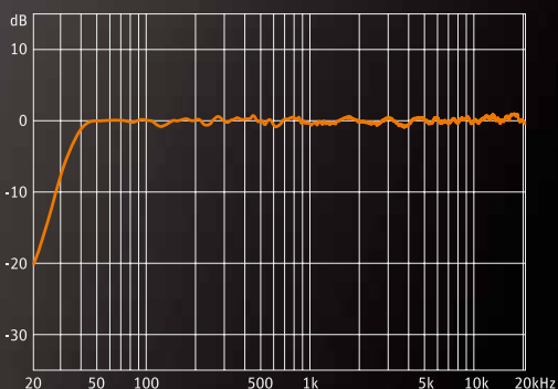
频率响应
